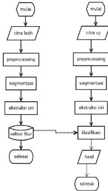
Gambar 4. Proses klasifikasi
